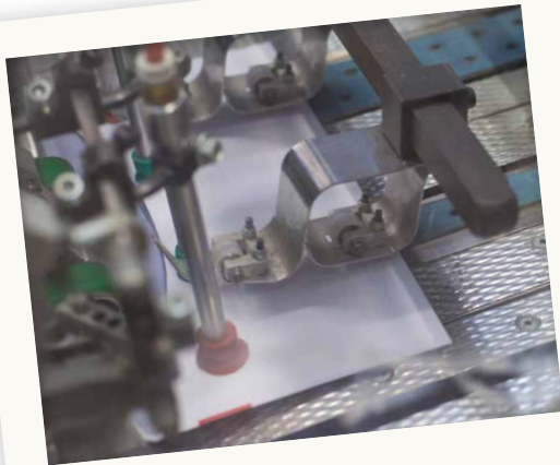
Kuvertierstraße Detail
